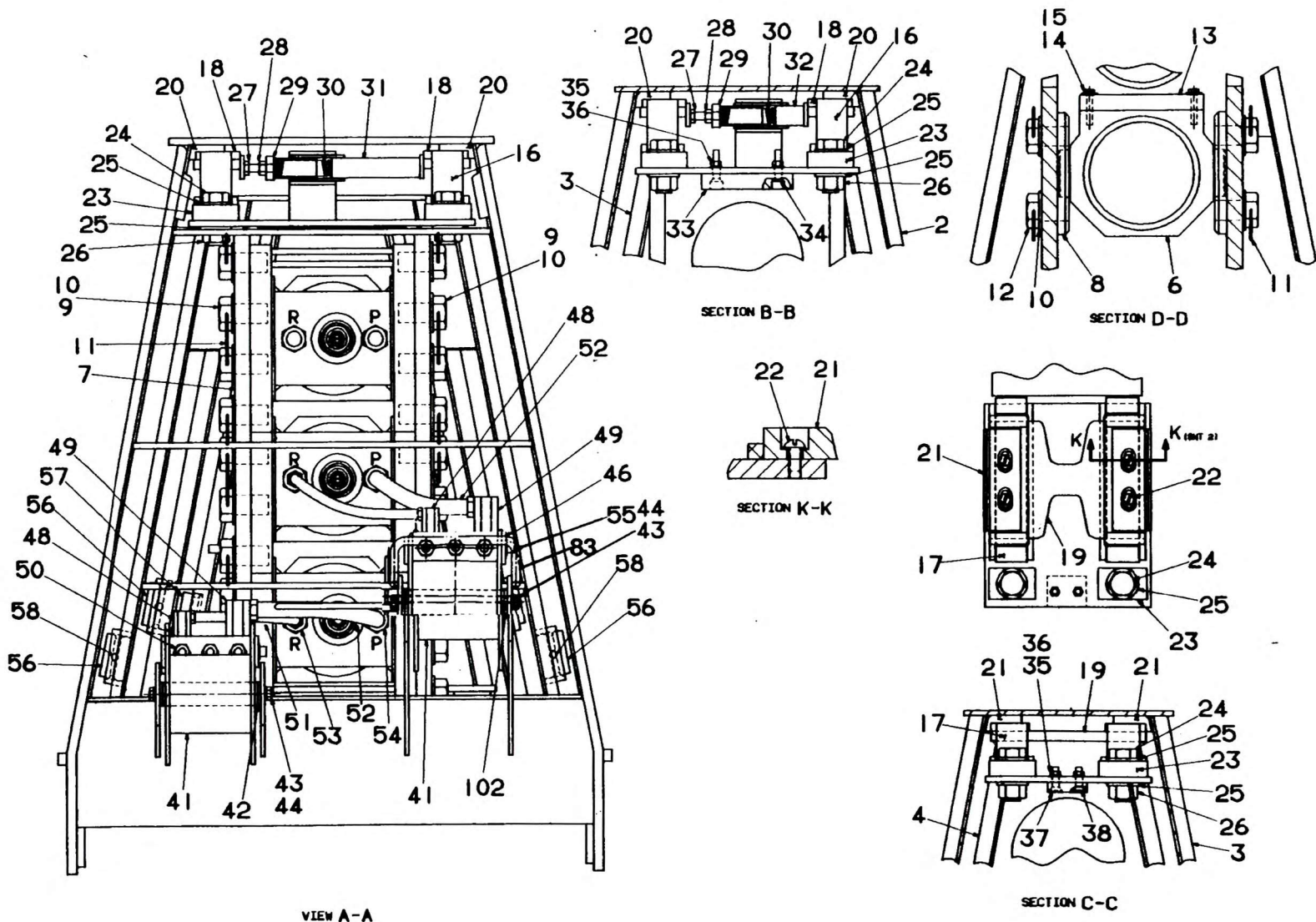
VIEW A-A
